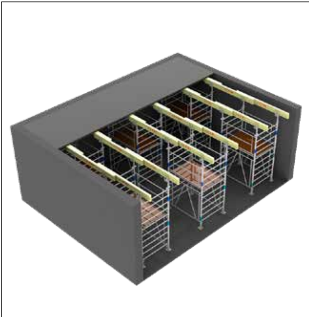
- Traggerüst für vorgefertigte Decken H20 auf Gerüstturm A120.
